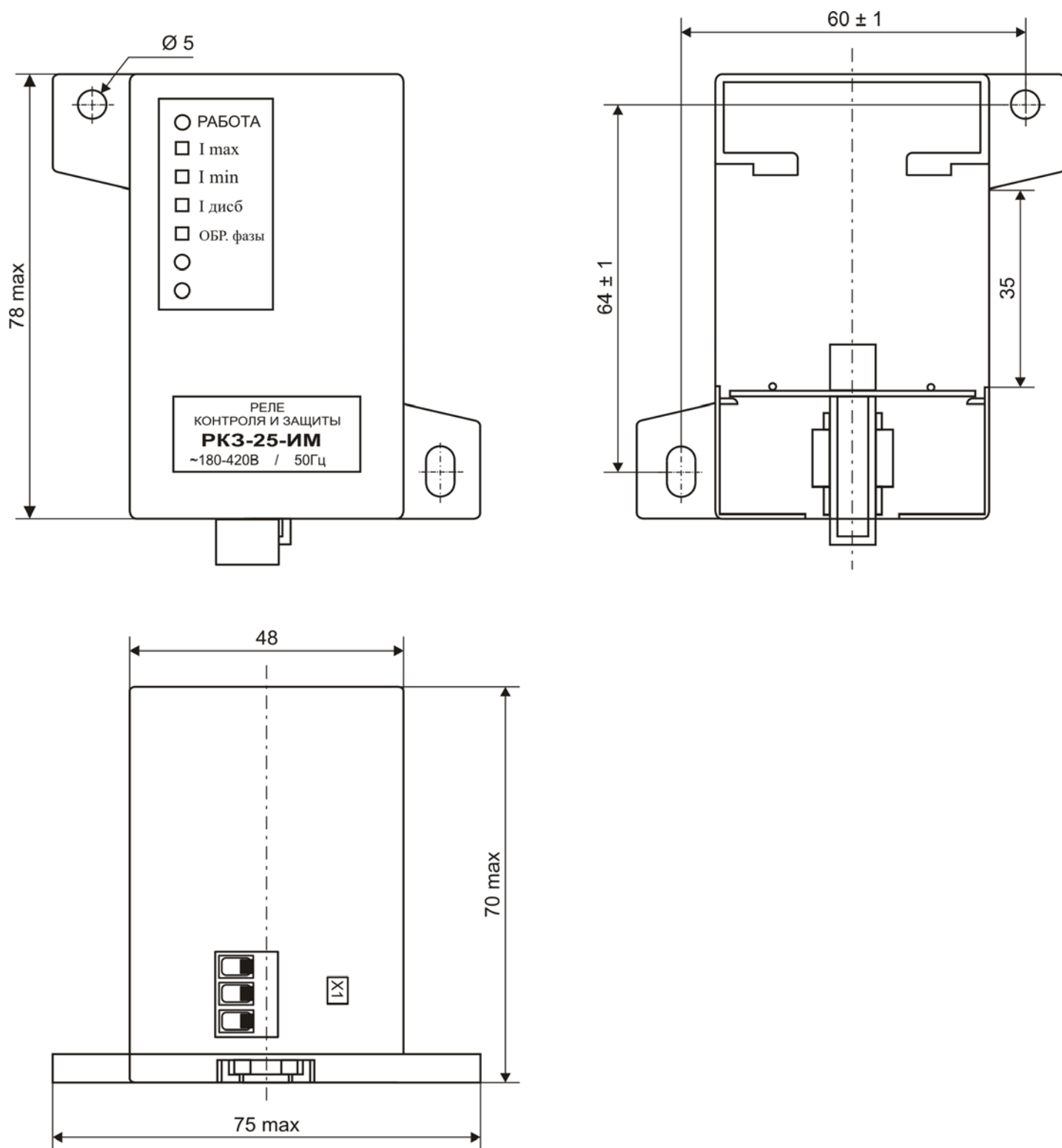
Рисунок 5 – Габаритные и установочные размеры реле
